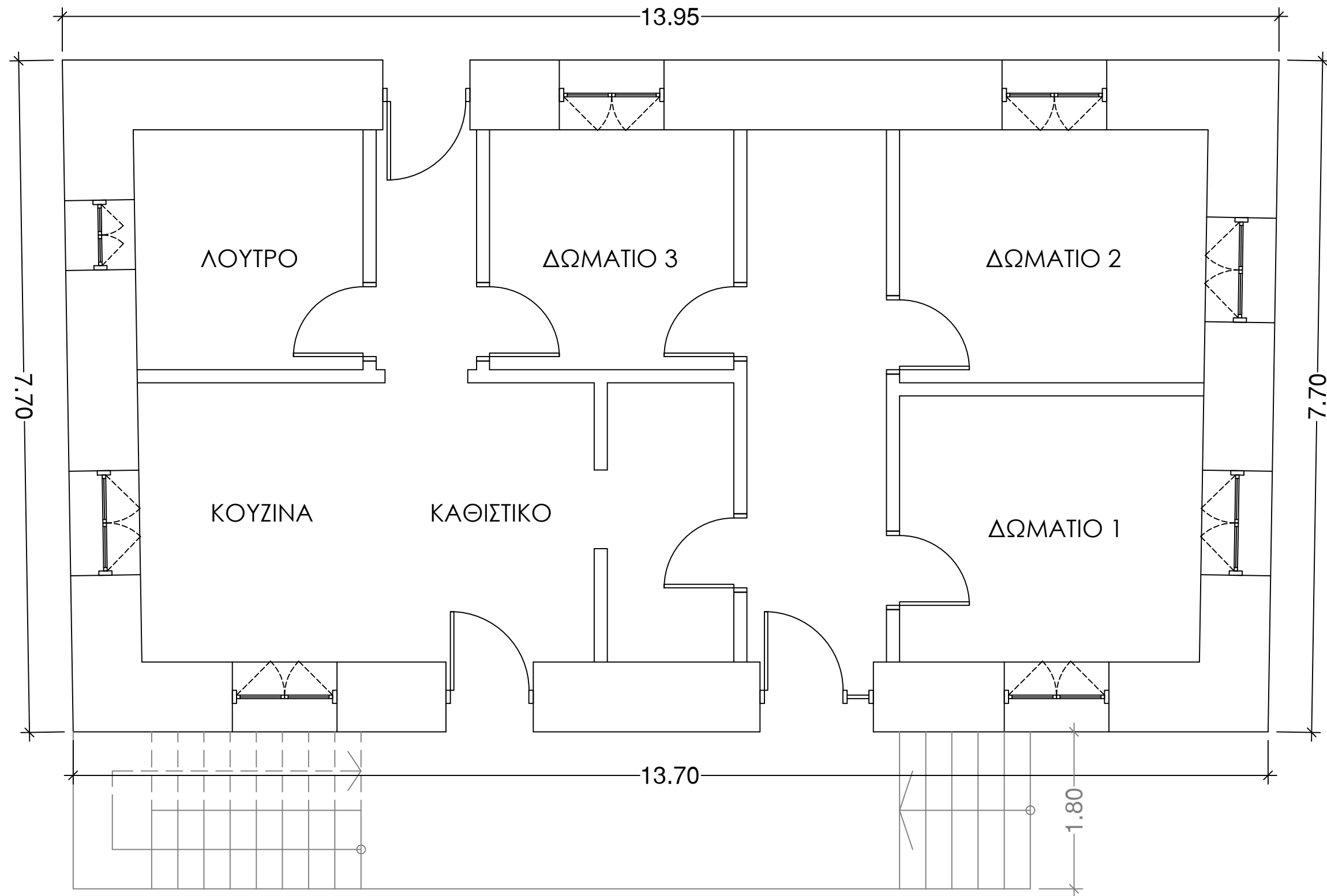
ΙΣΟΓΕΙΑ ΟΙΚΙΑ E=106.45m 2 (ΚΛΙΜΑΚΑ 1 : 50)
